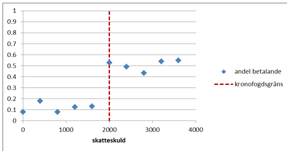
Figur 2 Grafisk illustration av RD-metoden baserat på påhittade data
